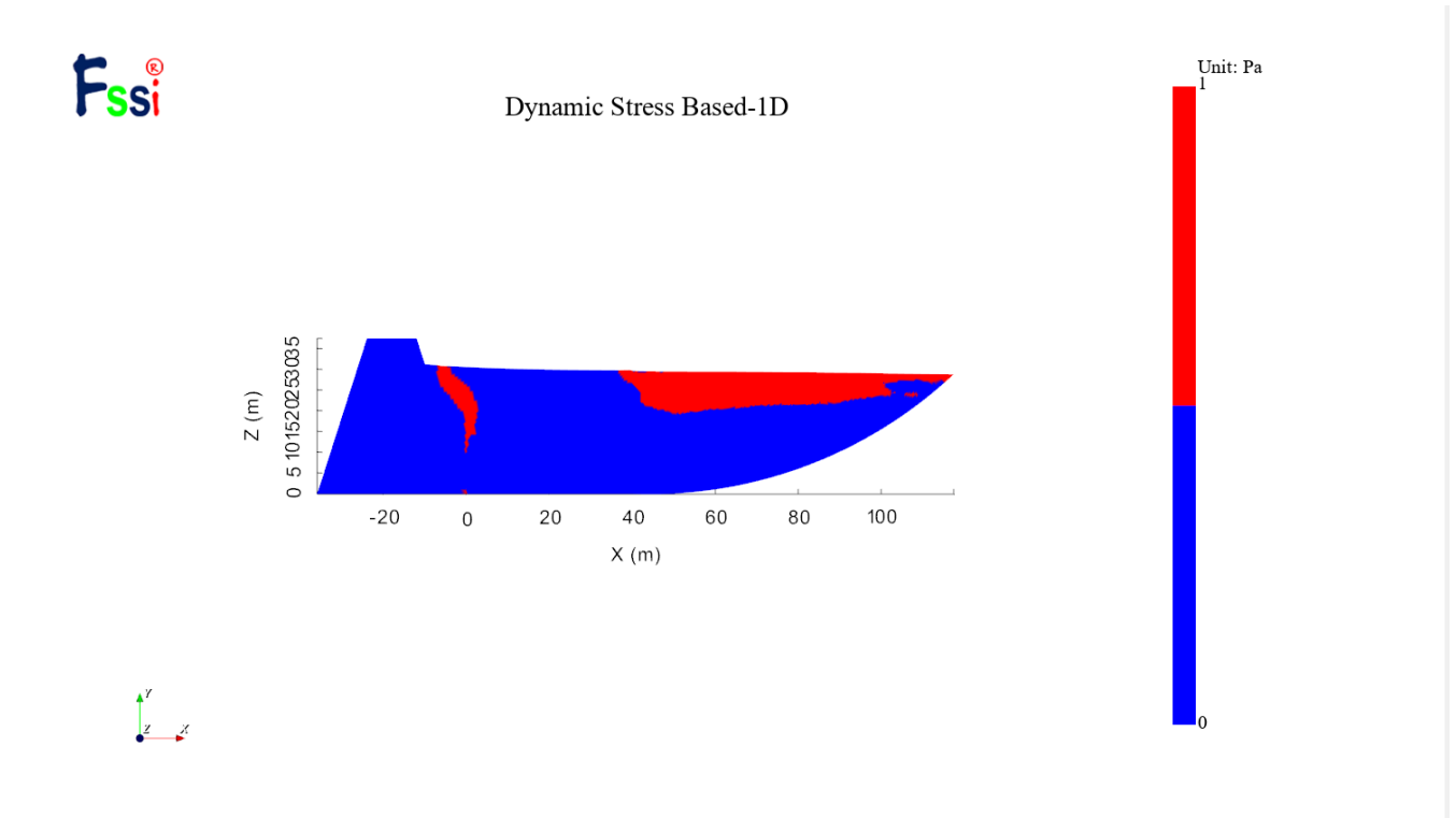
图 1-32 地震作用后(t = 22 s)液化区分布示意图
