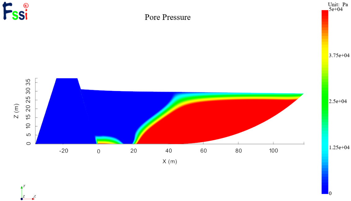
图 1-27 稳态渗流阶段( t = 2\text{ s} ) 孔隙压力分布图
