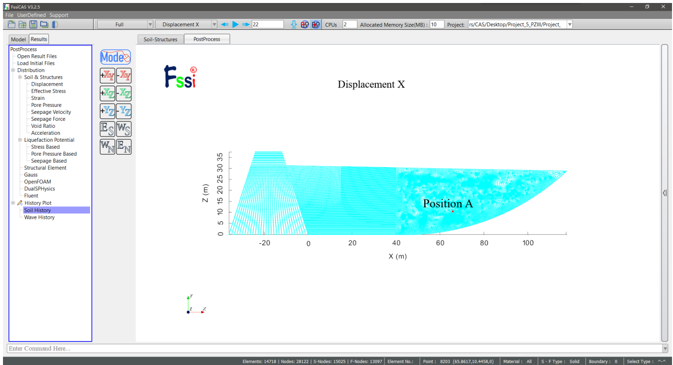
图 1-30 选择 No.8203 节点作为监测点 A 示意图
