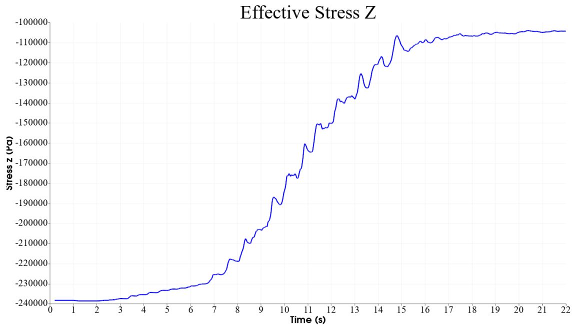
(b) Z 方向的有效应力时程曲线
