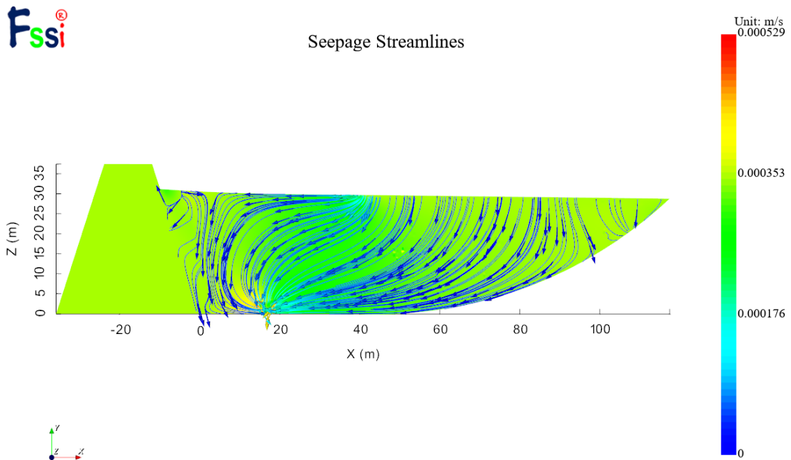
图 1-28 稳态渗流阶段( t = 2\text{ s} ) 时渗透流线分布图
