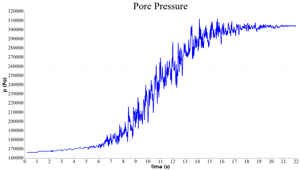
(a) 孔隙压力时程曲线
