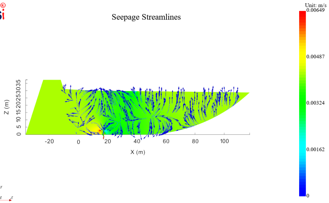
图 1-33 地震作用后( t = 22 s)的渗流流线分布图
